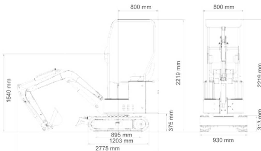
Schéma dimension HT10B
