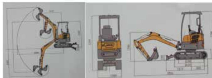
Schéma dimension HT20C
