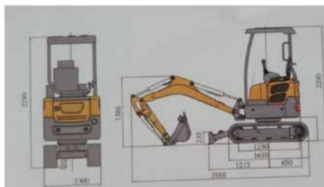
Schéma dimension HT25 classique
